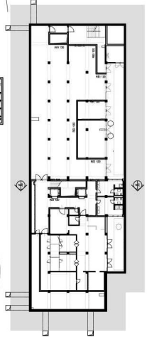
PIANTA PIANO INTERRATO 1:200
