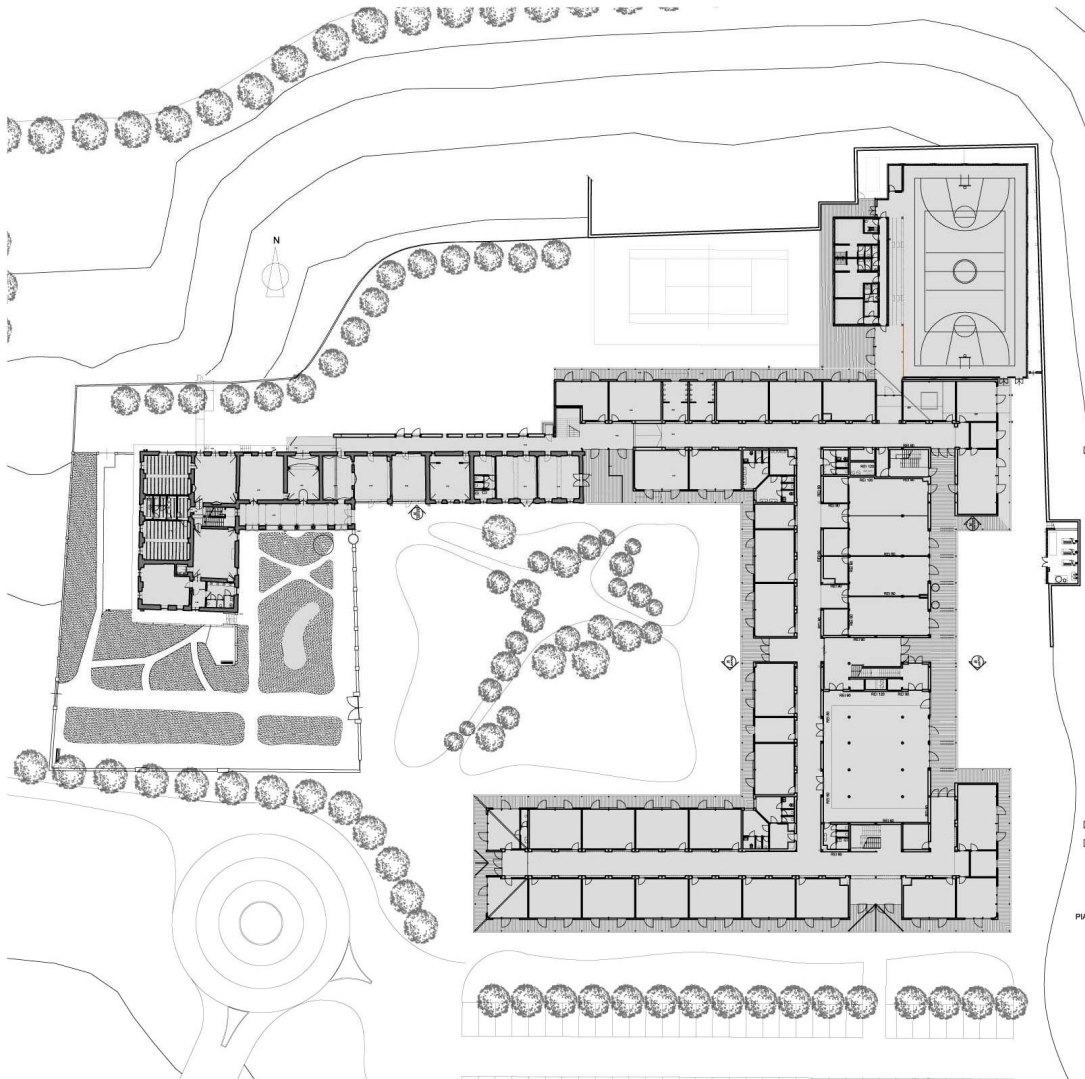
PIANTA PIANO TERRA 1:200
